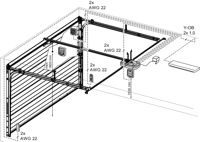
Abb. 3: Beispielinstallation Zubehör
